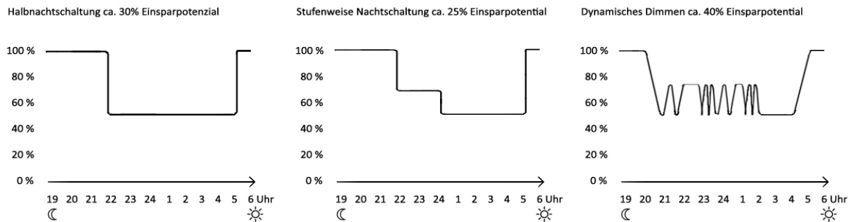
Abb. 10: Dimmvarianten: Halb- bzw. Stufenweise Nachtschaltung und flexible, sensorgestützte Steuerung, die sich am Verkehrsaufkommen orientiert, maximal 50% Dimmung zur Einhaltung der Norm.
